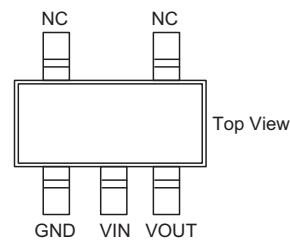
SOT23-5
