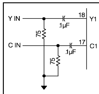
Fig. 6 - S-Video Input
