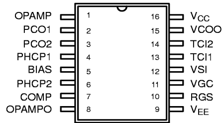
16 Pin SOIC
