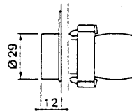
XB2-BA●● ZB2-BA●(1)
