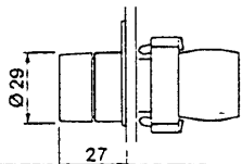
XB2-BD ●● ZB2-BD ●(1)
