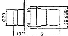
XB2-BW3.6. ZB2-BW1.8W3.,ZB2-BK... (1) ZB2-BW06.(2)
