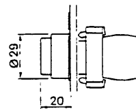
XB2-BL●● ZB2-BL●(1)
