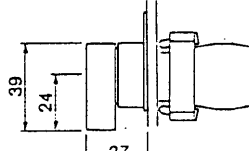
XB2-BJ ●● ZB2-BJ ●(1)
