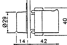
XB2-BV7 ● ZB2-BV0 ●(1) ZB2-BV7 (2)
