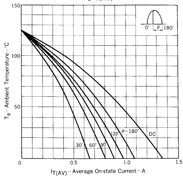
Fig. 11 T_a \cdot I_T(AV) RATING
