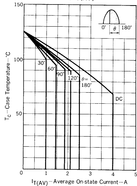
Fig. 10 T_C \cdot I_T(AV) RATING
