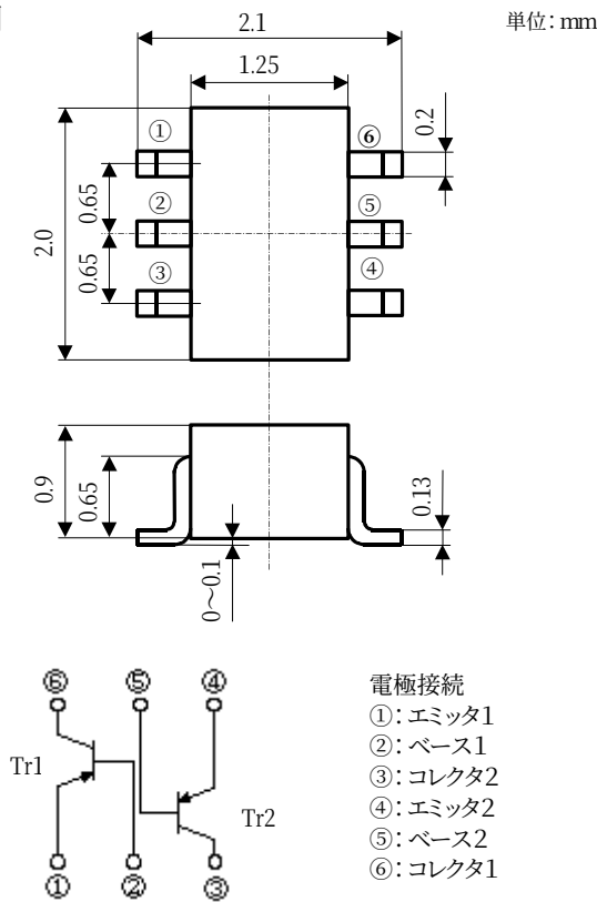
外形図
