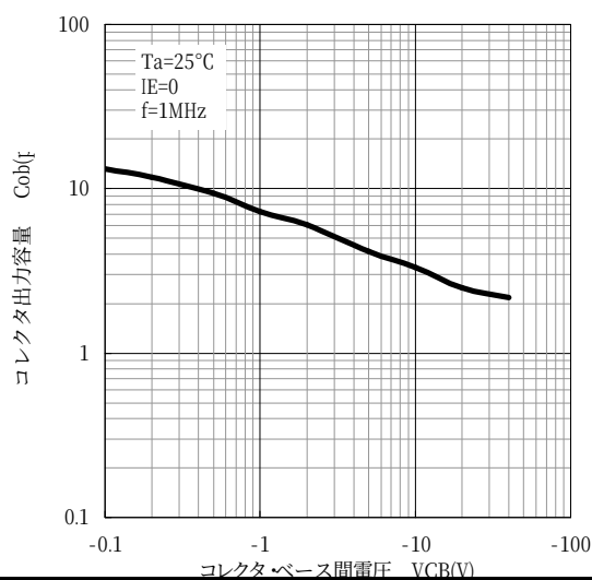
コレクタ出力容量 — コレクタ・ベース間電圧
