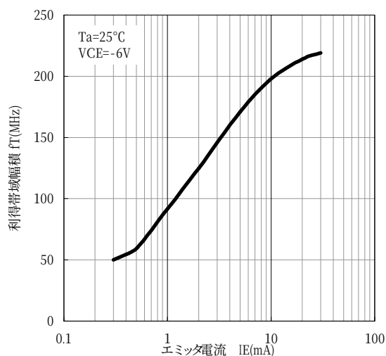
利得帯域幅積 — エミッタ電流
