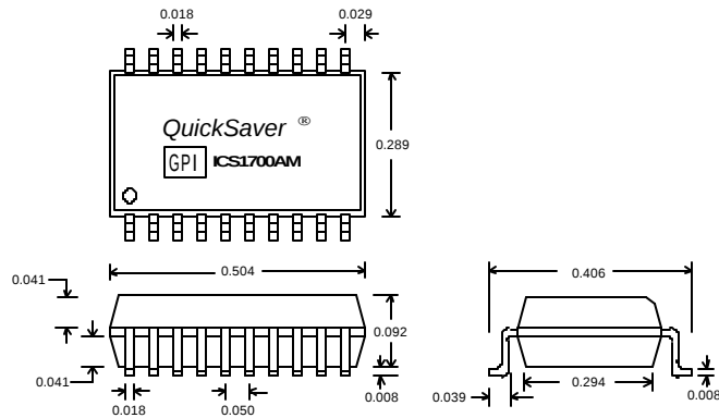
20-Pin SOIC Package (300 mil)
