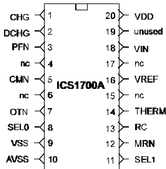
20-Pin SOIC
