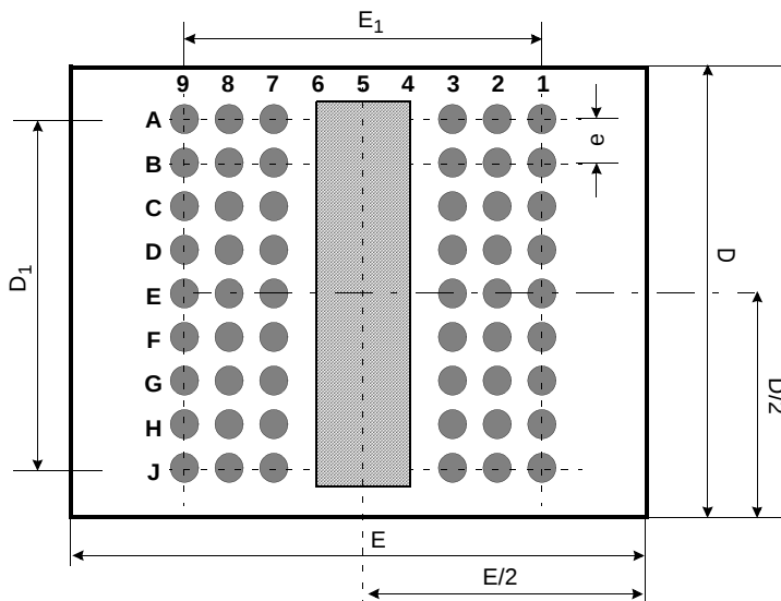
< Bottom View* 1 >
