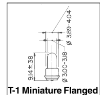
T-1 Miniature Flanged
