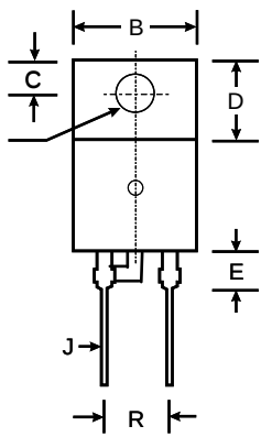
TO-220AC-P
