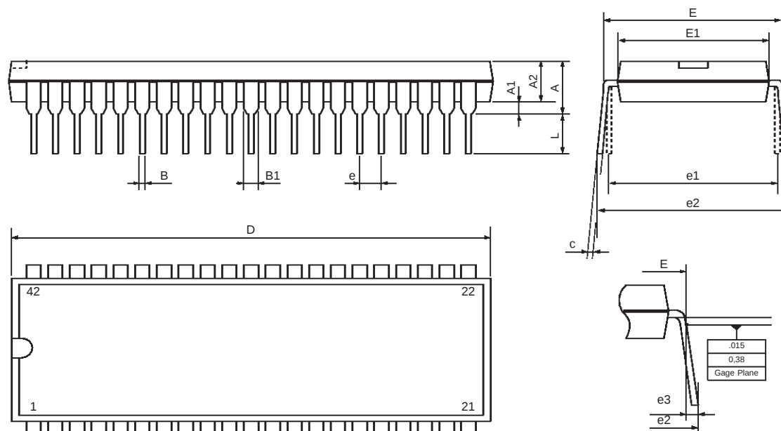
SDIP42
