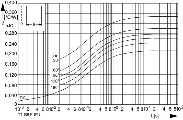
Bild / Fig. 20 Transienter innerer Wärmewiderstand je Zweig Z_{(th)JC} . Transient thermal impedance, junction to case, per arm Z_{(th)JC} .
