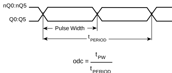
odc & t_{PERIOD}
