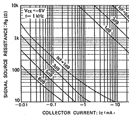
Fig.10 雑音特性 (I)
