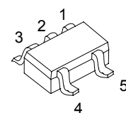
SOT-353
