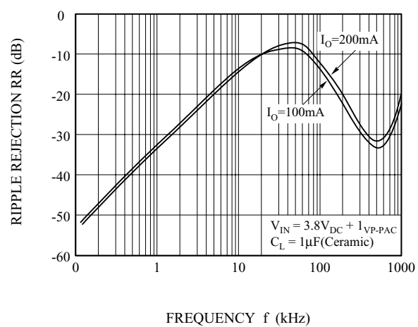
Fig. 8 PSRR
