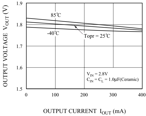
Fig. 1 I_{OUT} - V_{OUT}
