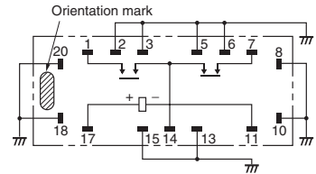
G6WU-1P
