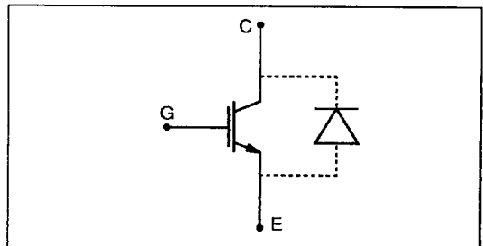
Fig.2 ITE08X06 circuit
