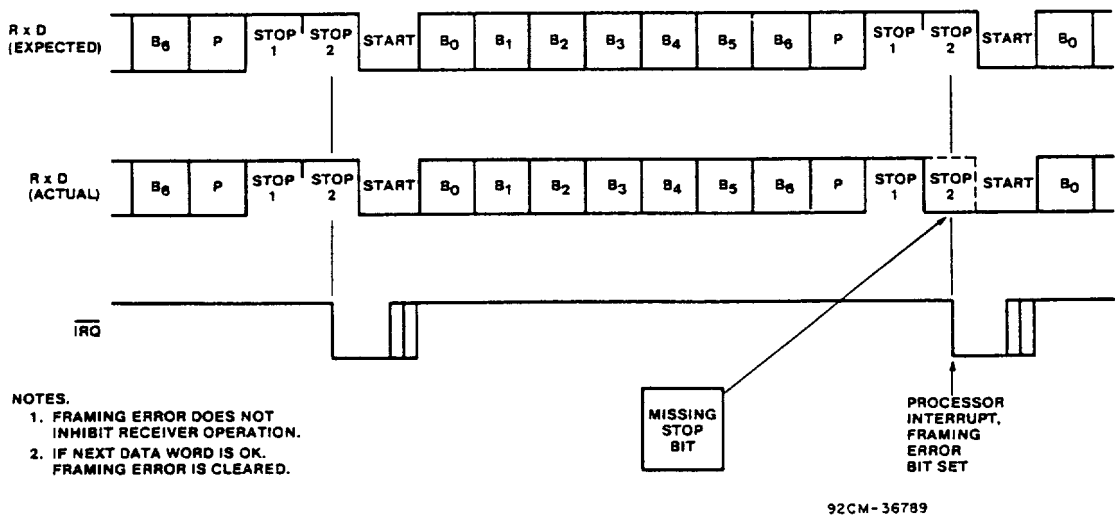
Fig. 15 - Framing error.
