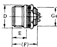
Bulkhead Receptacle
