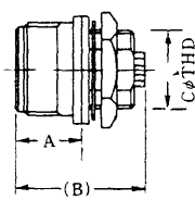
Bulkhead Receptacle
