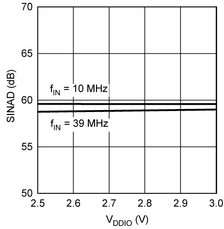
SINAD vs. V_{DDIO}
